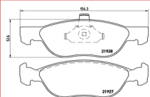
Pastiglia anteriore
