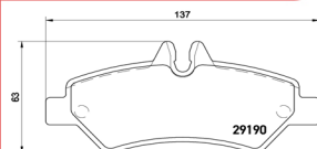
Pastiglia posteriore
