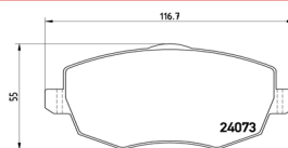
Pastiglia anteriore
