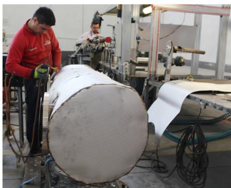
SILENZIATORE DI SCARICO PER BARCA/ PER NAVE
