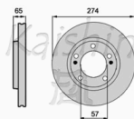
Disco freno Posteriore
